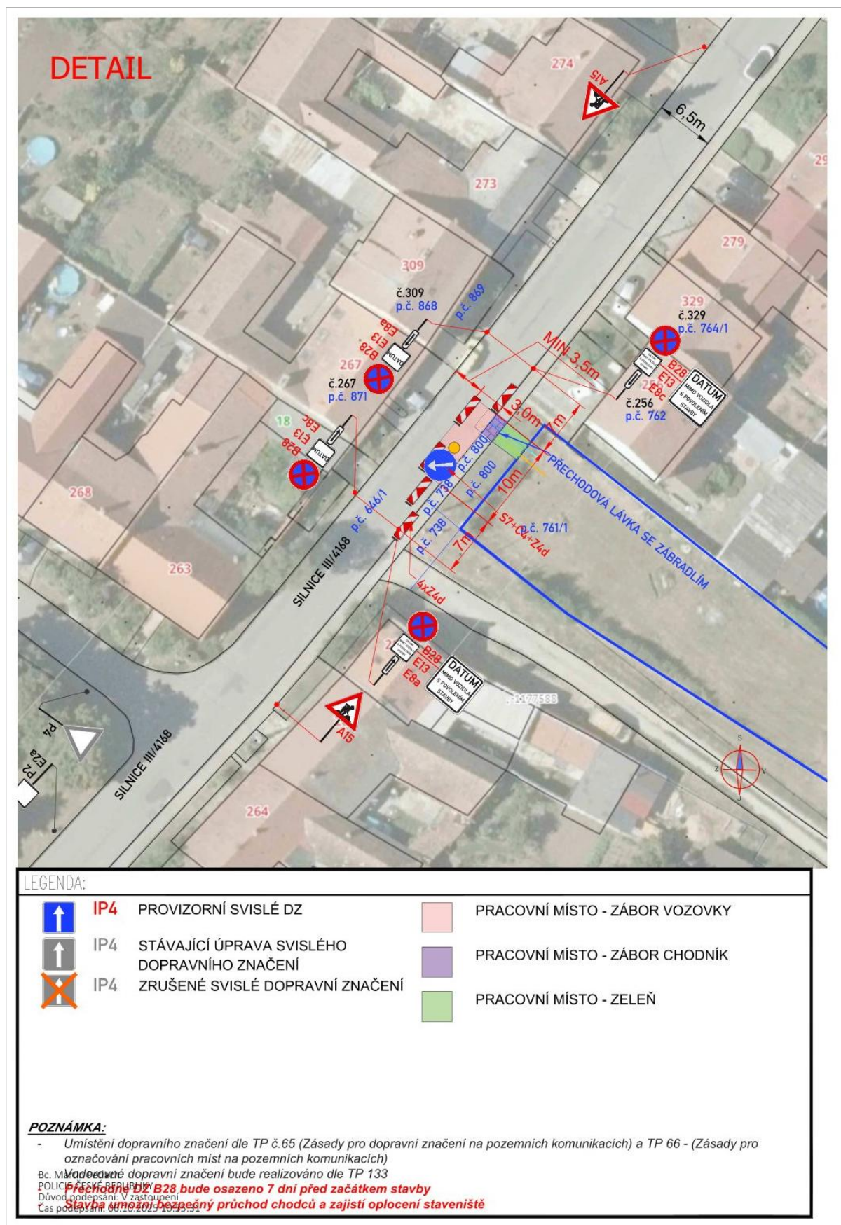
Obázek 1 – situace dopravního značení
